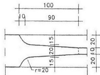
SEZIONE ORIZZONTALE SULLA RASTREMAZIONE
