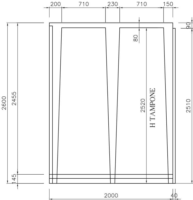
VISTA LATERALE
