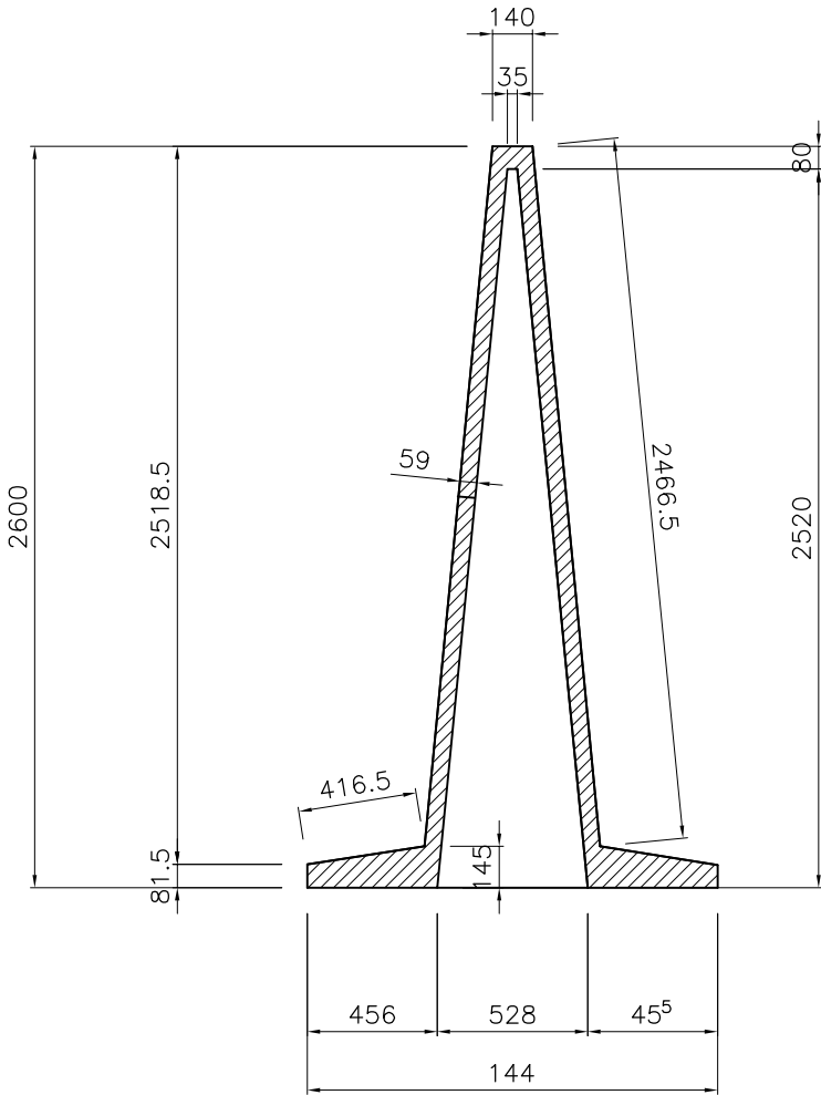
SEZIONE IN CORRISPONDENZA DEL TAMPONE
